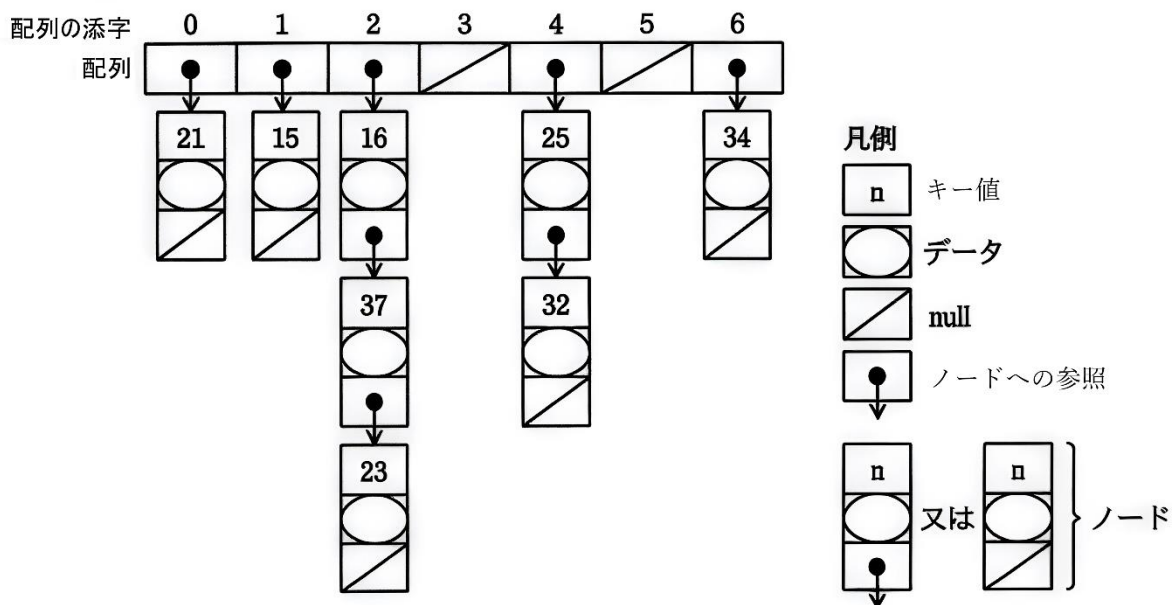
図1 チェイン法のデータ格納例
