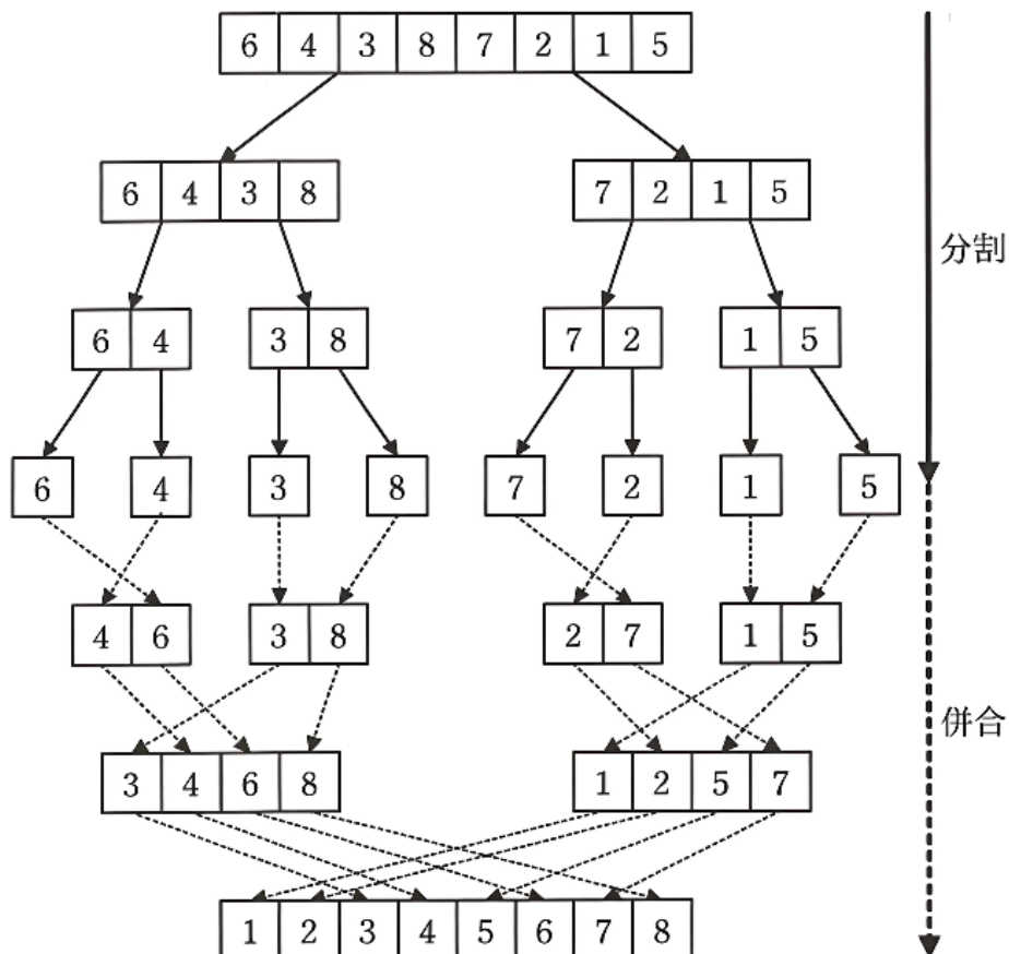
図 1 アルゴリズムの流れ
