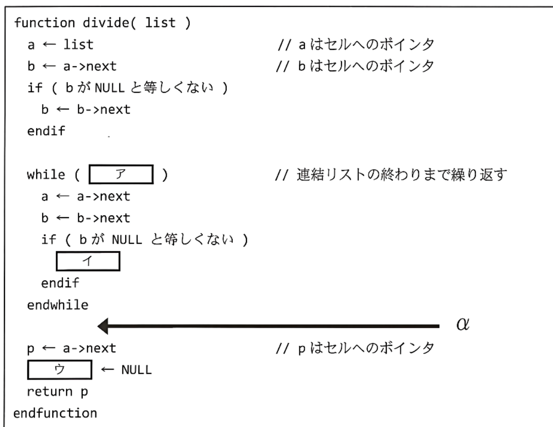
図 5 関数 divide のプログラム
