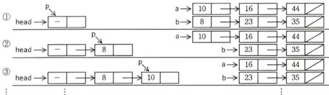
図 6 連結リストの併合の流れ
