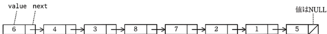
図 3 連結リストのデータ構造
