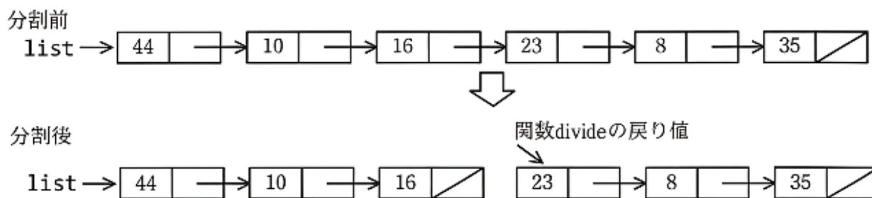
図 4 連結リストの分割前後のイメージ
