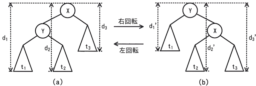
図 4 木の回転の様子
