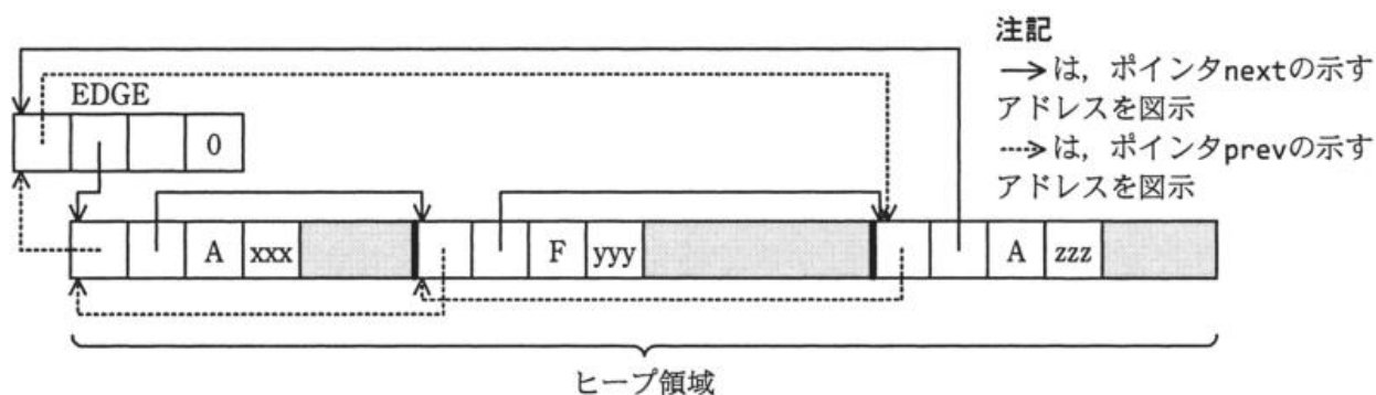
図2 メモリ管理のためのデータ構造
