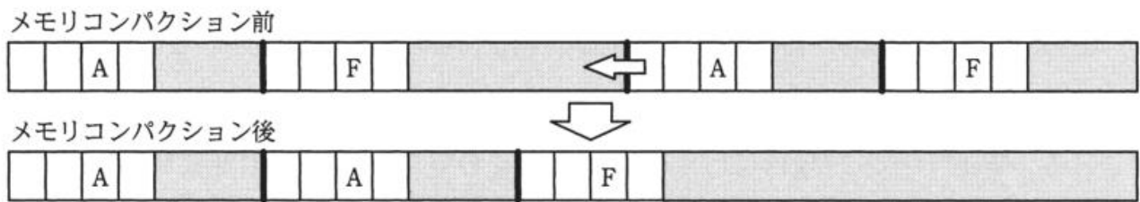
図 5 メモリコンパクションのイメージ
