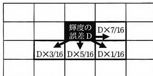
図 2 拡散先の数 4 の場合の、誤差拡散のパターンの例
