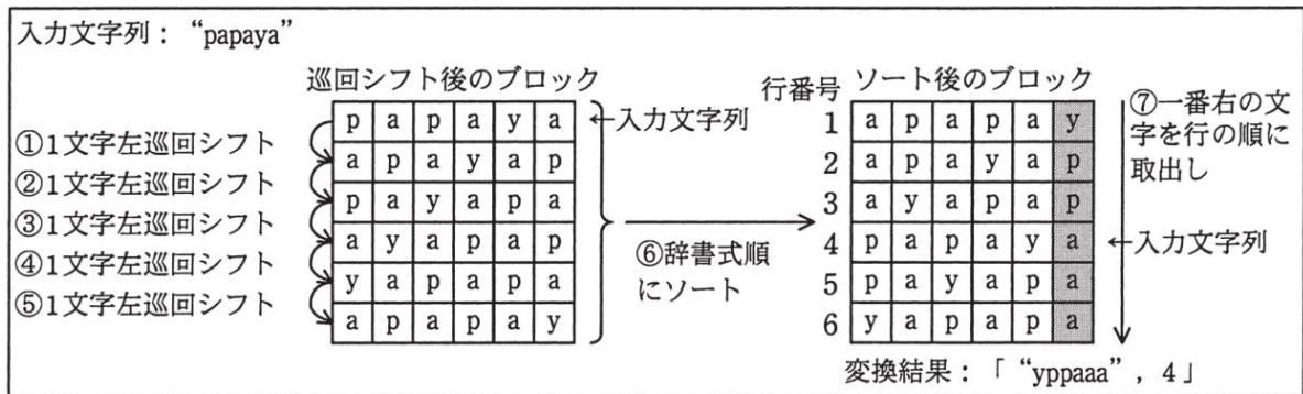
図 2 Block-sorting の変換処理
