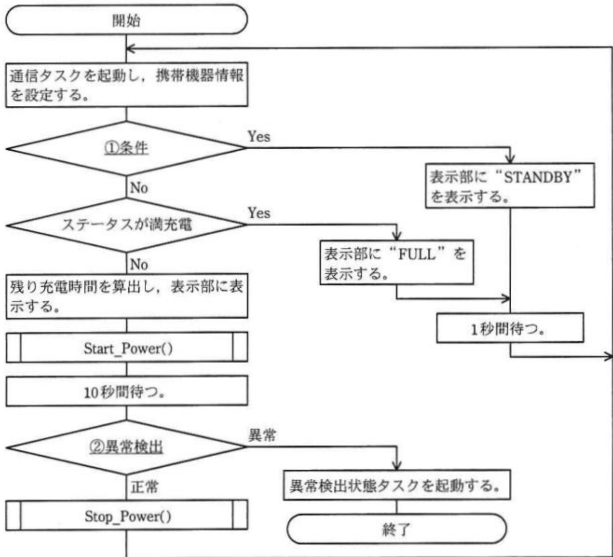
図 2 メインタスク処理の流れ図
