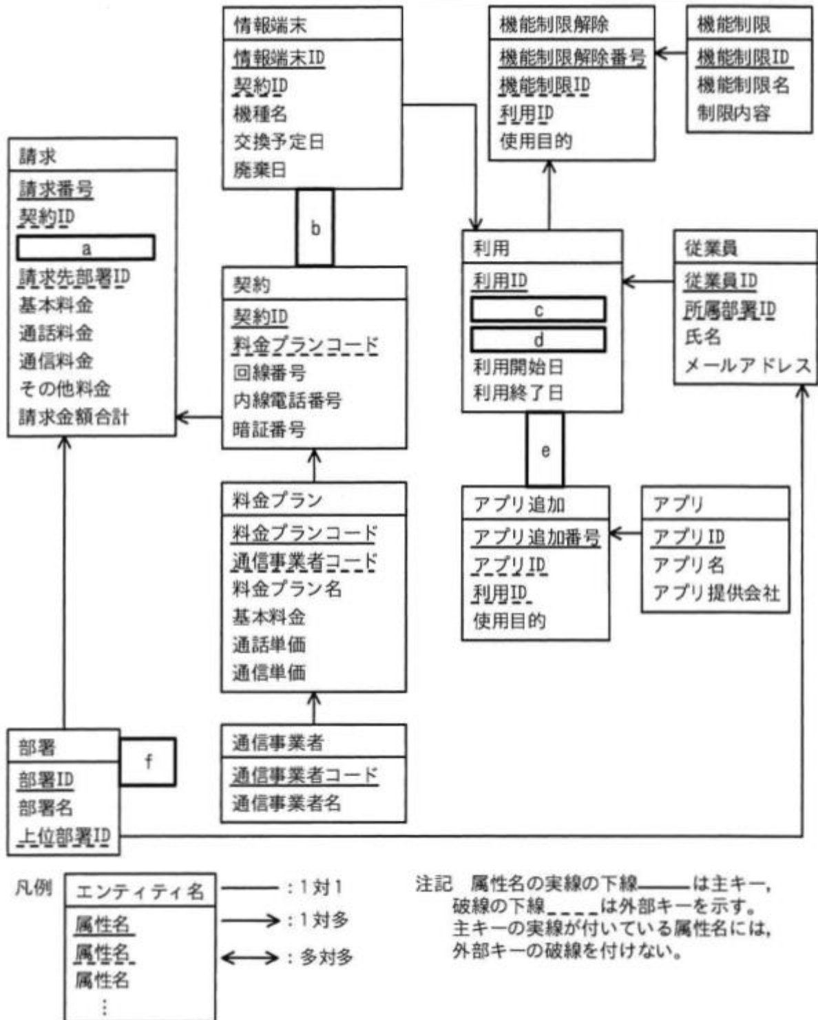
図 1 新システムの E-R 図 (抜粋)
